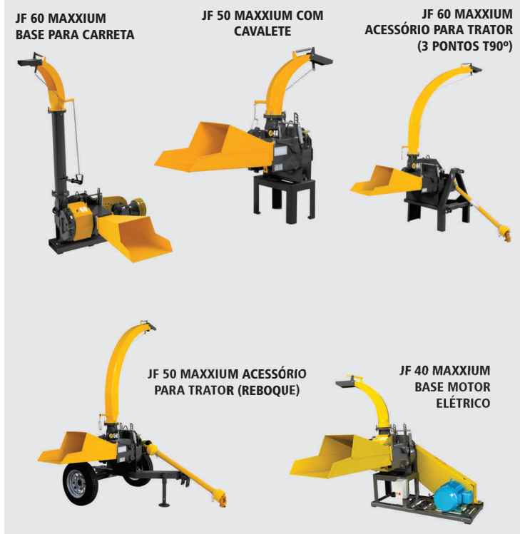
TRANSMISSÃO COM CAIXA DIRETA NO ROTOR Para JF 50 e 60 Maxxiium nas versões com acessórios para reboque, trator 3 pontos (T90°) e base para carreta.
